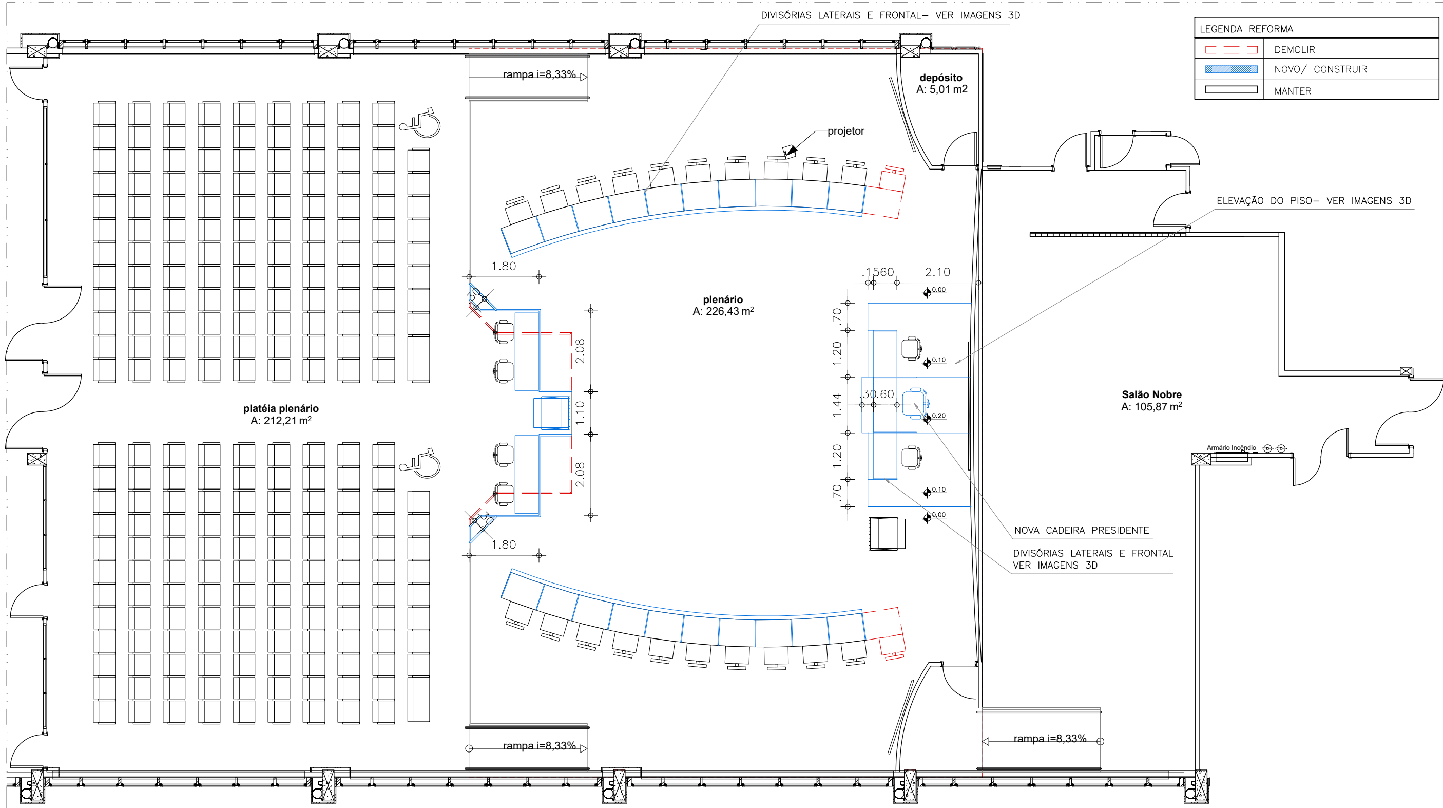
PLANTA REFORMA ESC 1/100
