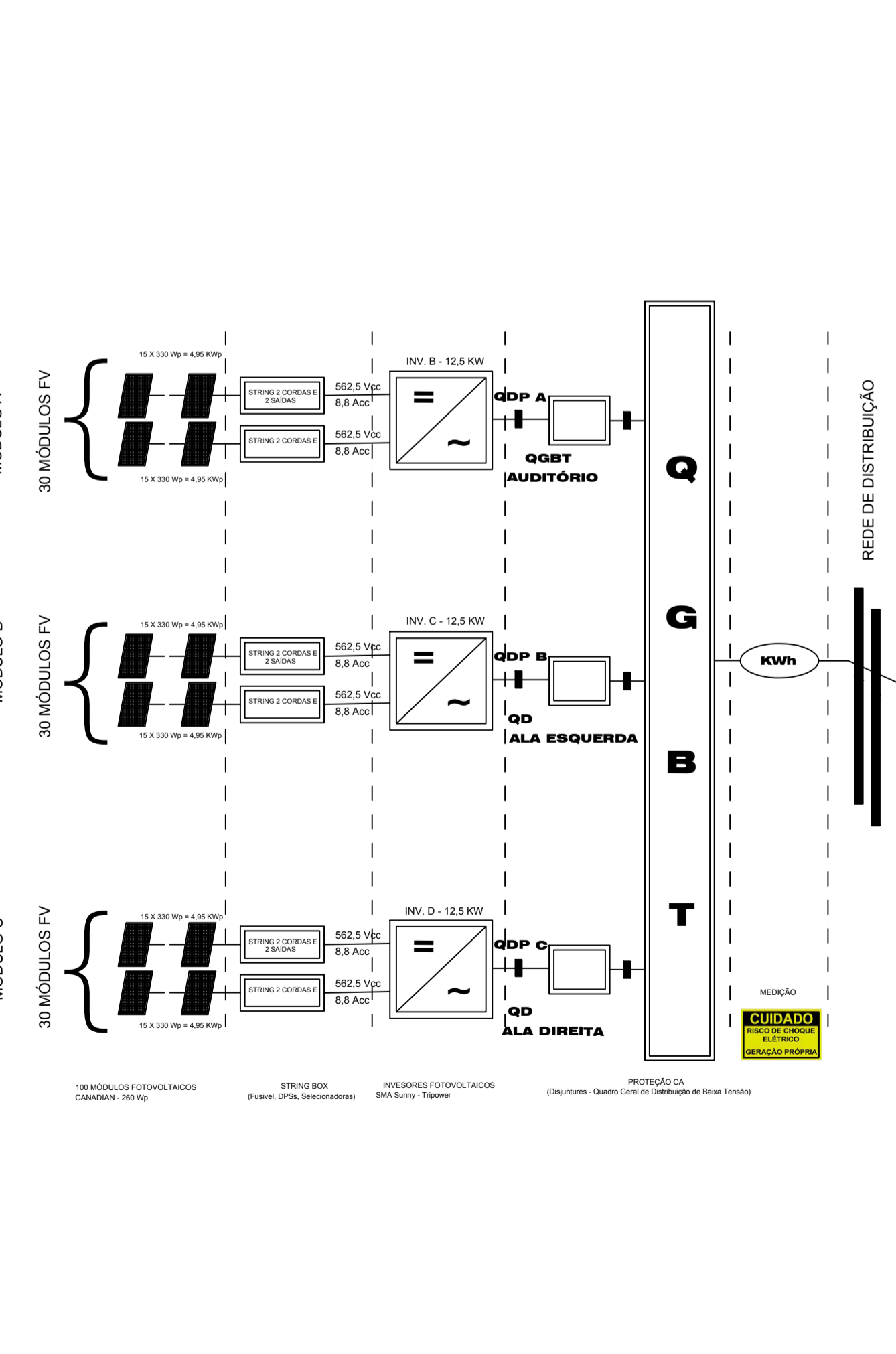
02 ESTRUTURA DE CONEXÃO A SER ADOTADA ESCALA: S/E
