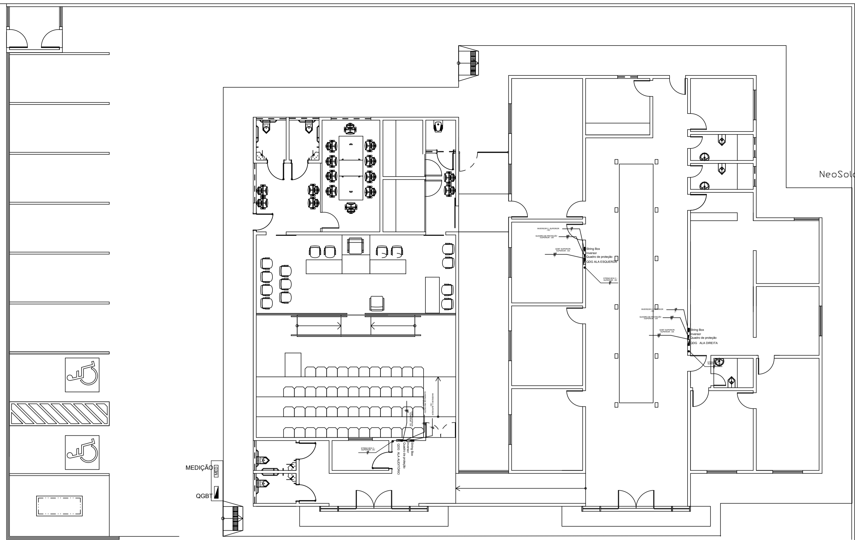
01 PLANTA DE LOCALIZAÇÃO DOS QUADROS FOTOVOLTAICOS ESCALA: 1/100
