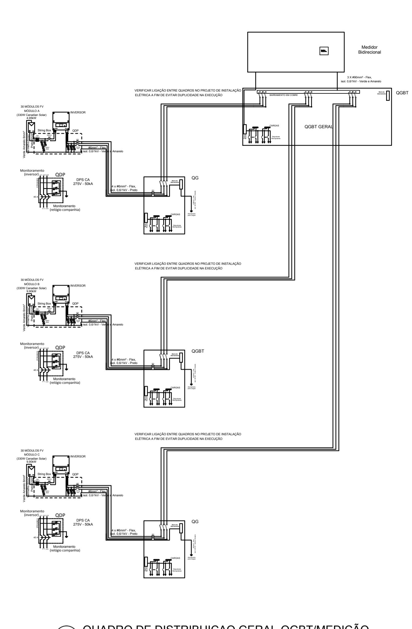
03 QUADRO DE DISTRIBUIÇÃO GERAL-QGBT/MEDIÇÃO SEM ESCALA
