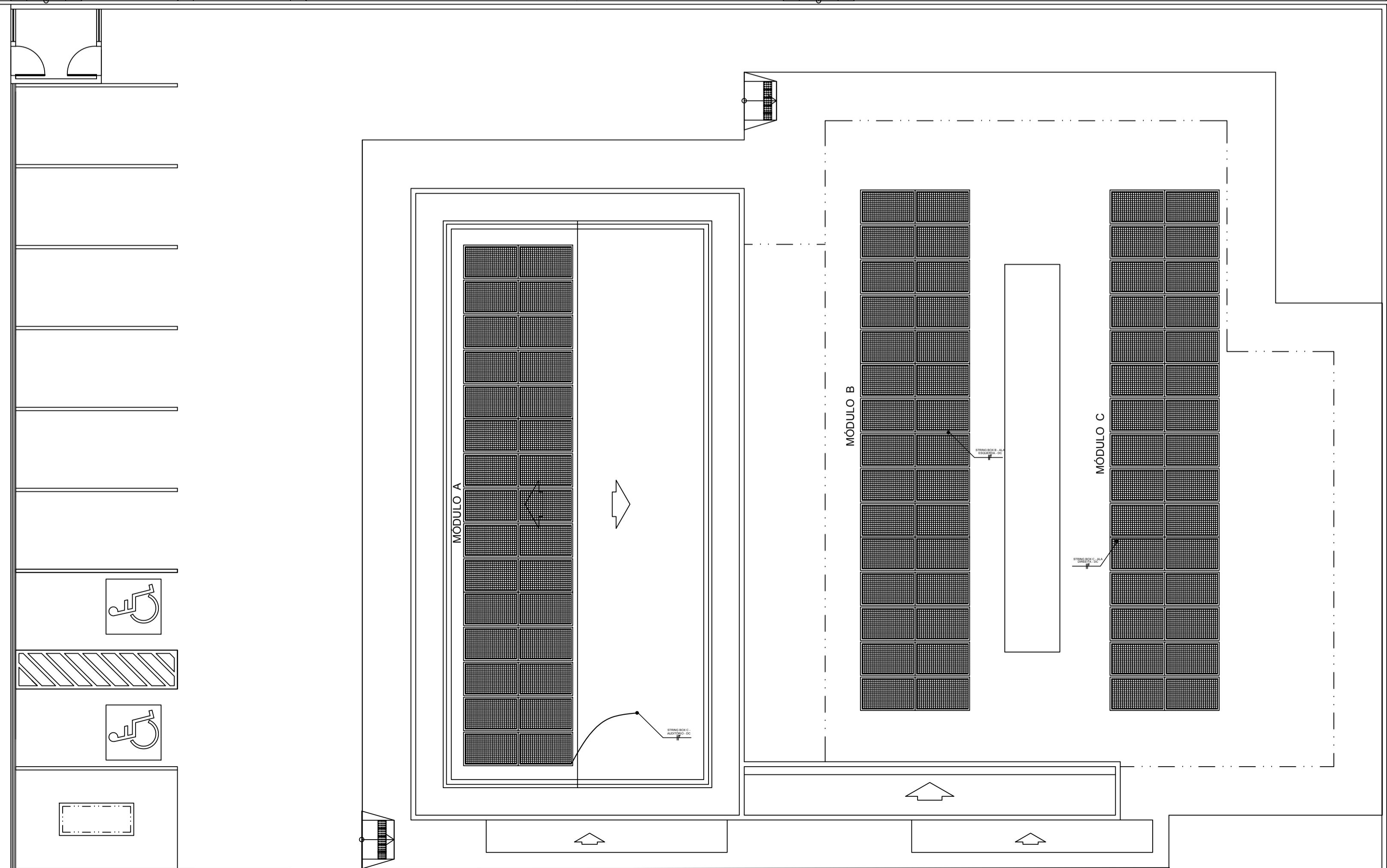
01 PLANTA DE LOCALIZAÇÃO DE MÓDULOS FOTOVOLTAICOS ESCALA: 1/100
