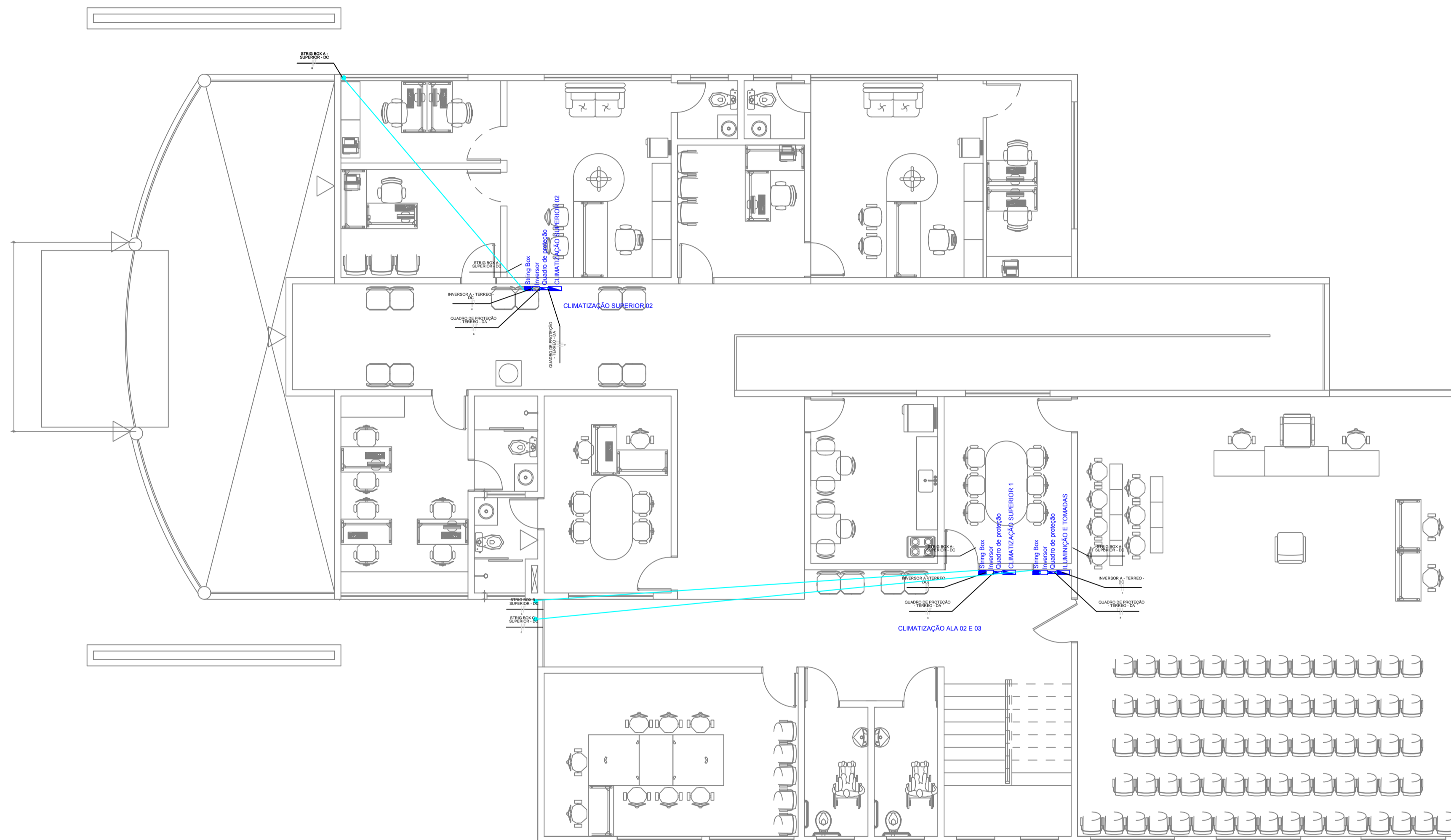
01 LIGAÇÃO NO PAVIMENTO TERREO ESCALA: 1/75
