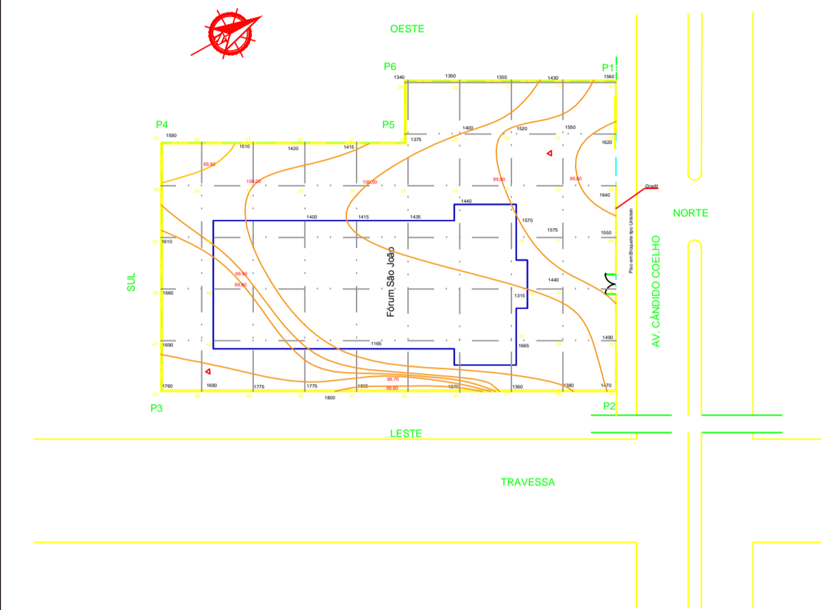
03 PLANTA DE LOCALIZAÇÃO ESCALA: 1/500
