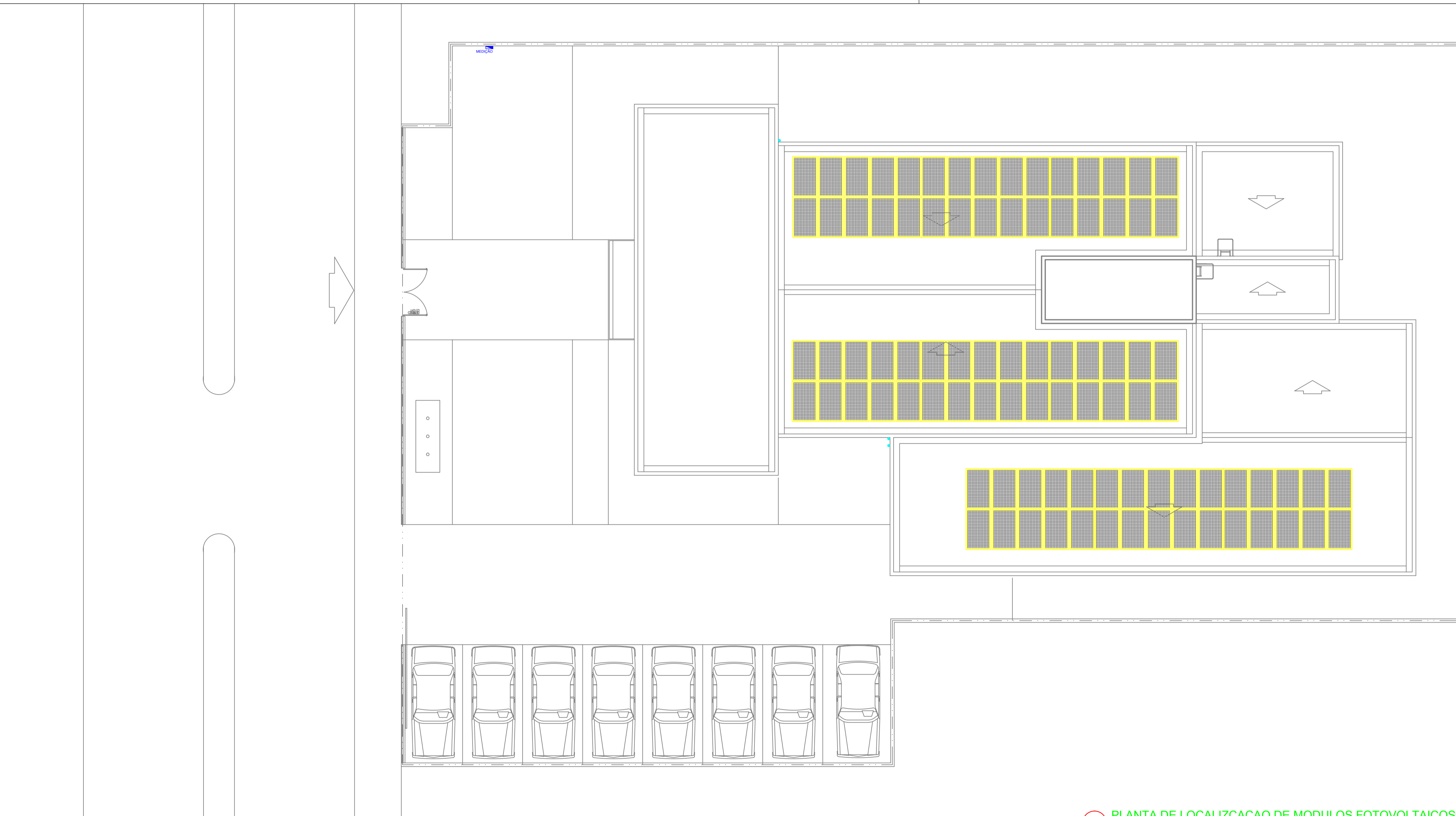
05 PLANTA DE LOCALIZAÇÃO DE MÓDULOS FOTOVOLTAICOS ESCALA: 1/100
