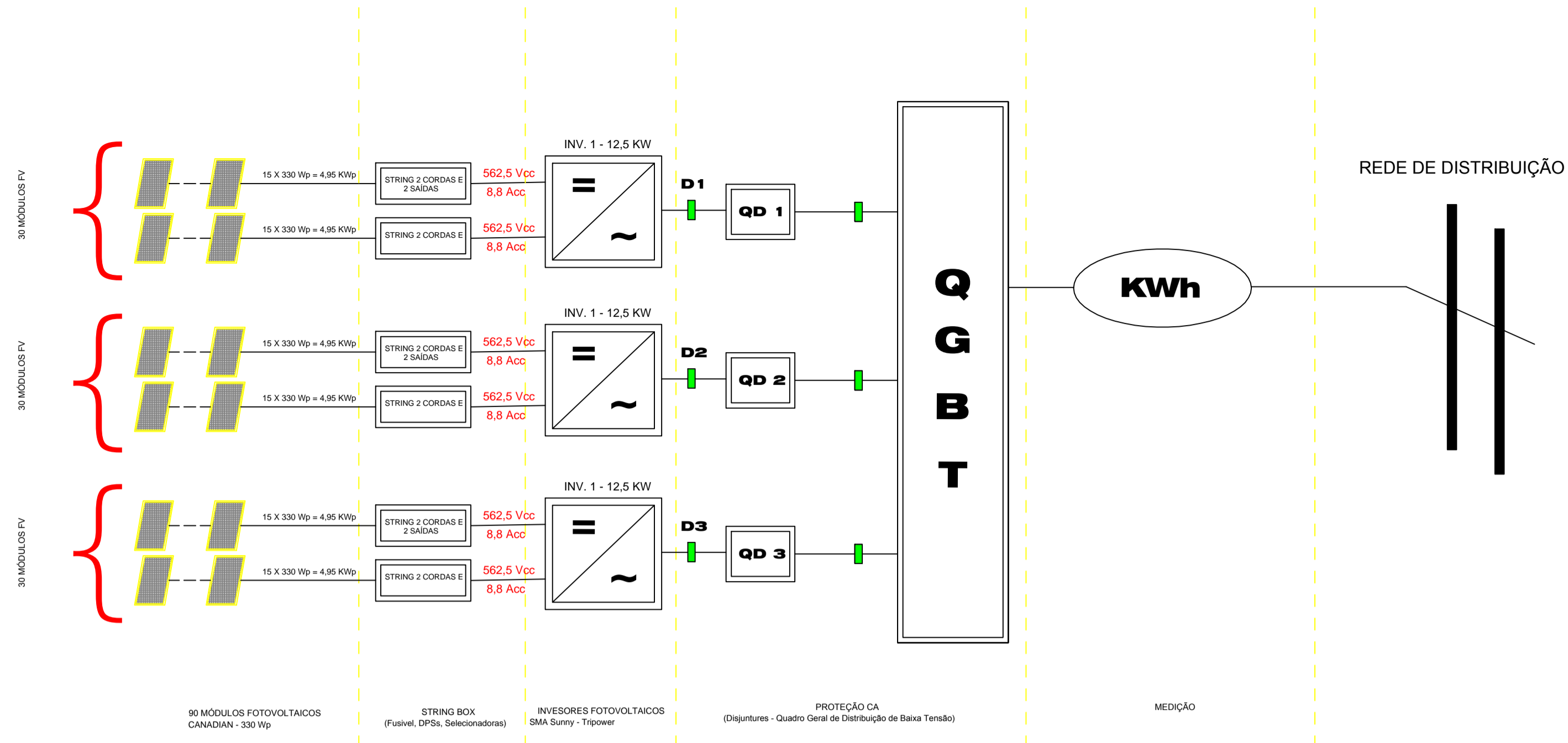
02 ESTRUTURA DE CONEXÃO A SER ADOTADA ESCALA: S/E
