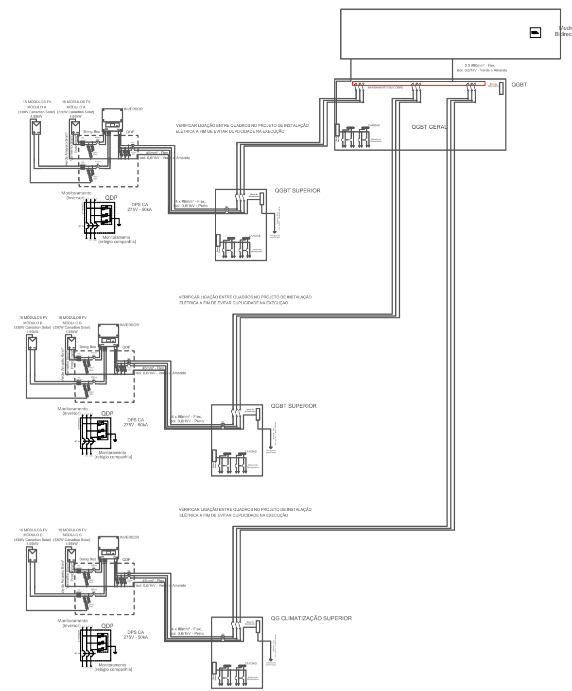
03 ESTRUTURA DE LIGAÇÃO COM O SISTEMA FOTOVOLTAICO ESCALA: S/E
