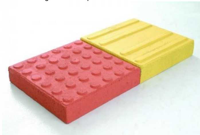
Figura 45: Piso podotátil em concreto.
