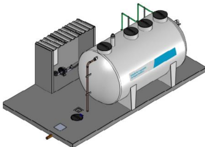
Figura 2: Modelo do sistema da ETE Compacta
