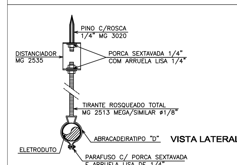
04 DETALHE DE FIXAÇÃO DE ELETRODUTO SEM ESCALA DEFINIDA
