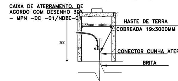
DET. DO ATERRAMENTO
