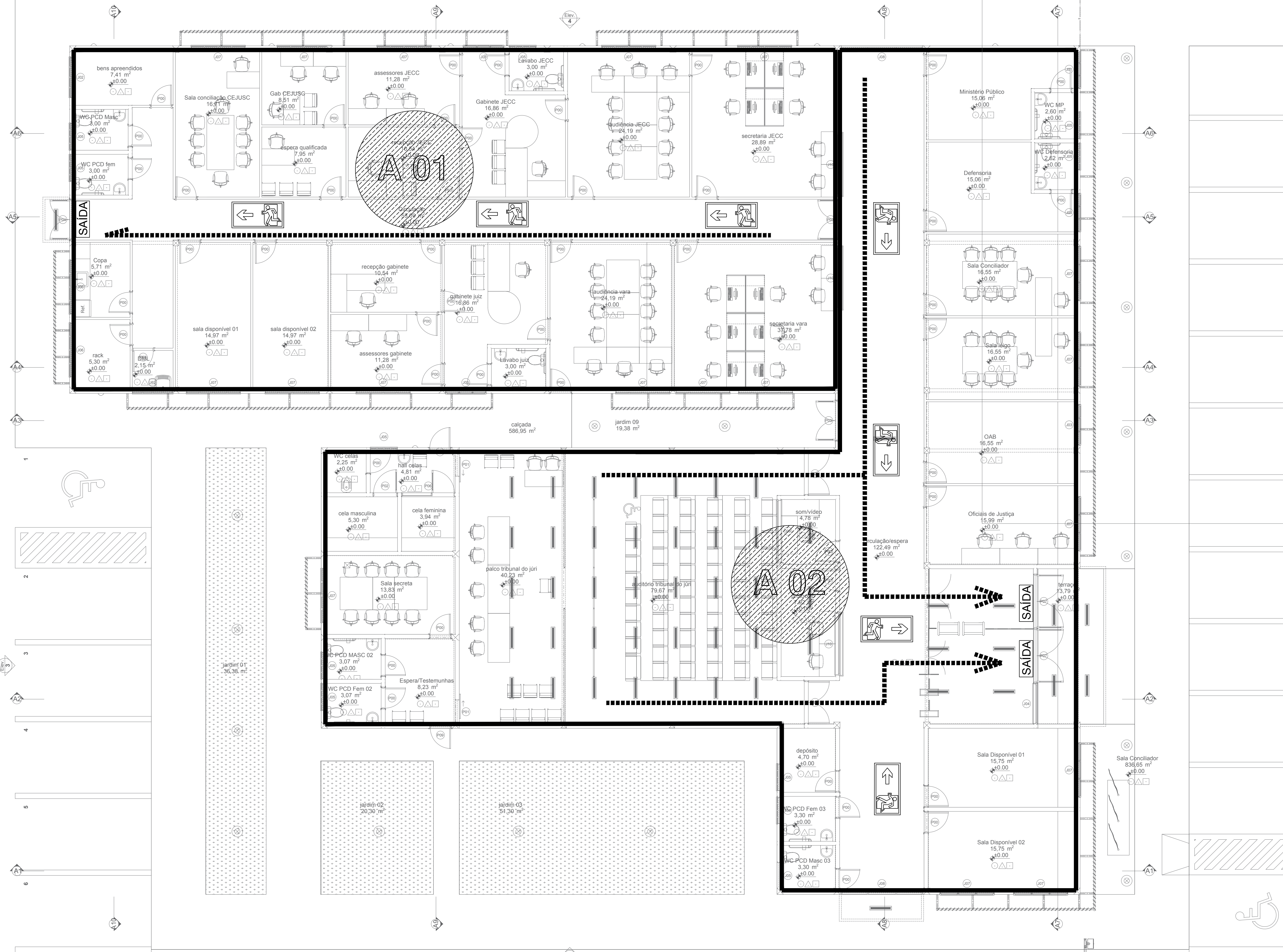
PLANTA SETORES
